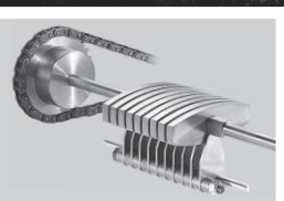
Pelletsbrenner mit patentiertem Drehrost für optimale Verbrennung
